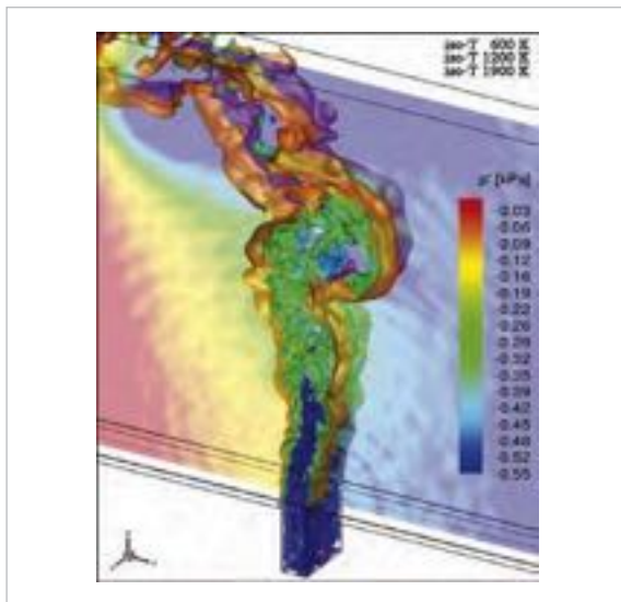
Simulazione LES di fiamma premiscelata CH 4 /H 2 /Aria
