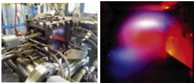
Bruciatore sperimentale Trapped Vortex ENEA per turbine a gas
