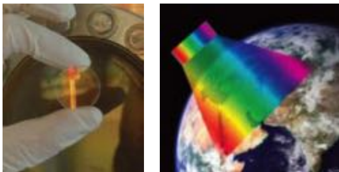
Filtri ottici variabili per strumentazione dedicata all'osservazione della Terra
